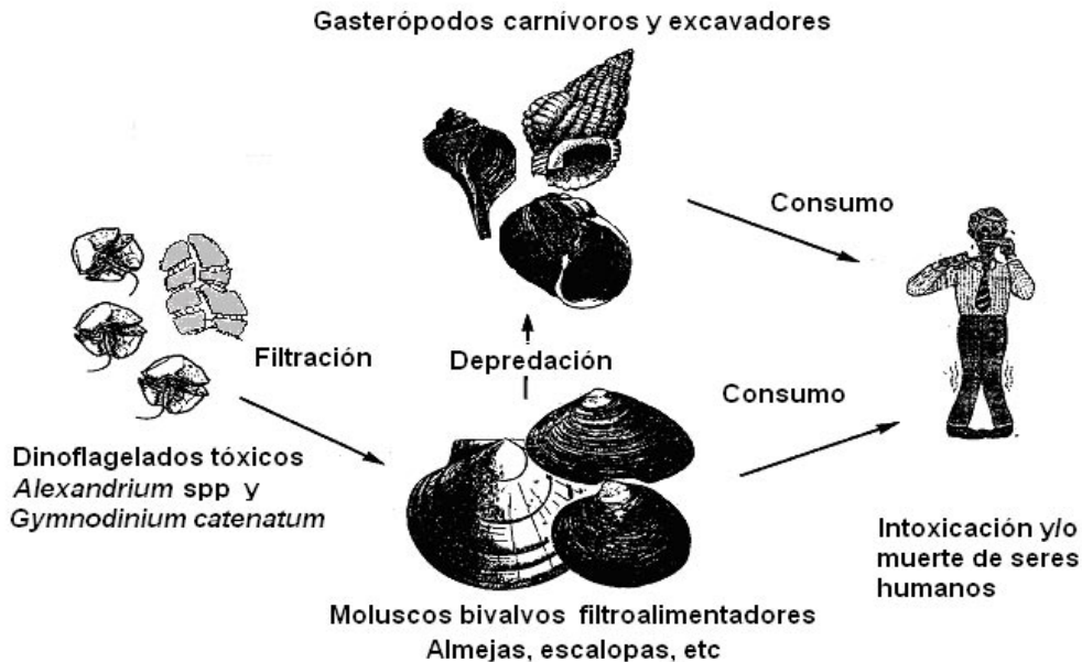
Figura 1.- Escenario que ilustra como las toxinas paralizantes pueden ser acumuladas por los moluscos, llegan a causar la intoxicación de los seres humanos. (Modificado de 34).
